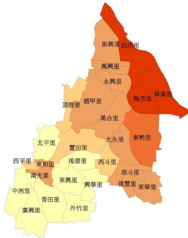
圖 1-3-4 土壤液化分布圖
